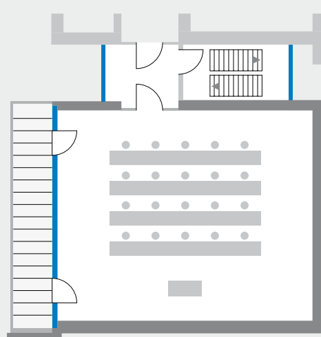
Grundriss OG Seminar-, und Arbeitsräume
